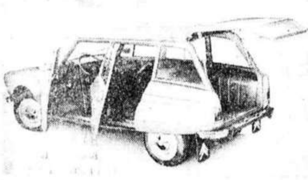
CITROËN AMI 8 BREAK Motor: 2-sylindret, luftkjolet, 602 ccm. HK: SAE 35, DIN 32, ved 5750 omdr./min. Forhjulsdraft, 4-dørs. Registrert for 4 personer. Lengde: 3,99 m, bredde: 1,52 m, bagasjerom: 330 liter, vekt, kjøreklar 725 kg. Akselerasjon: 0-80 ikke oppgitt, 0-100 ikke oppgitt. Toppfart: 120 km/t. Pris fra kr. 25 750.
