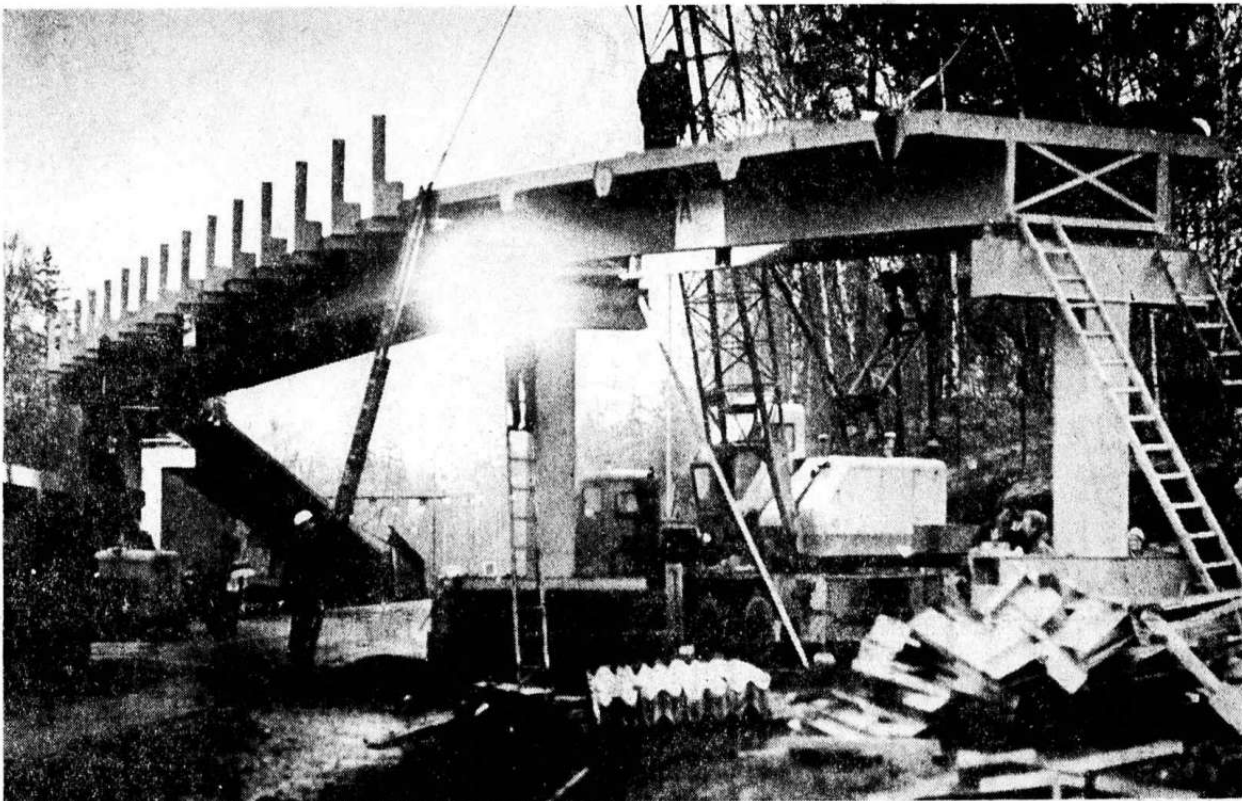
Den midlertidige bro over Fornebu-krysset er en helt ny type i Norge, og det finnes neppe maken i Skandinavia. Det er en såkalt elementbro — satt sammen av stålplater, 130 meter lang.
